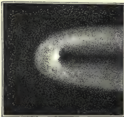
September 22. (Pepe.)
